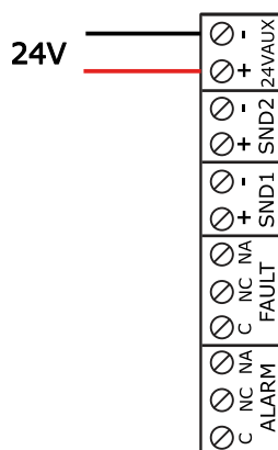
Figura 15 Collegamento di uscita ausiliaria a 24 V
