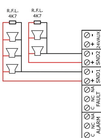
Figura 14 Cablaggio dell'uscita della sirena
