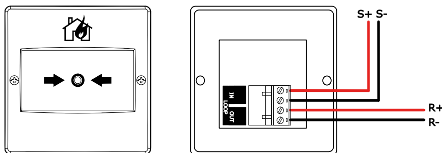
Figura 20 Dettaglio del cablaggio di un pulsante di allarme analogico
