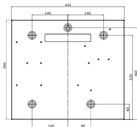
Figura 6 Dimensioni per il montaggio della scatola a parete
