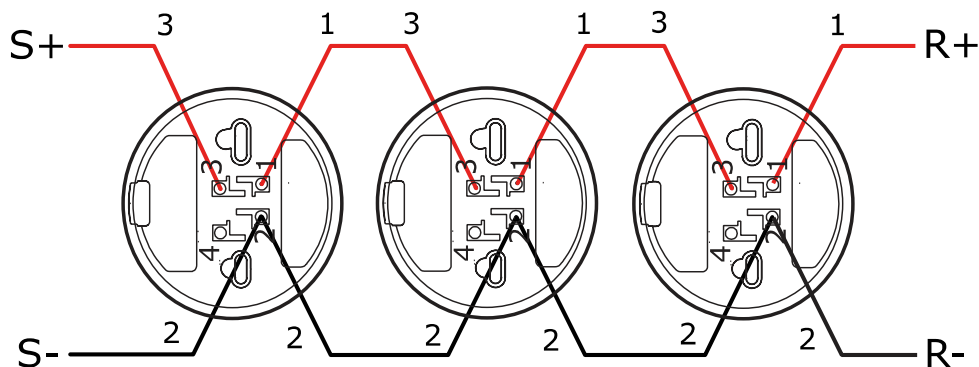
Figura 17 Collegamento di un circuito analogico con rivelatori a isolatore
